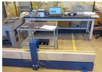
Testovací pracoviště se senzorovým systémem první generace v prostorách ÚJV Řež, a. s.
